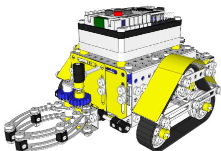
Obrázek 6.10: ME - Robotické pásové vozidlo s diferenciálně řízeným podvozkem
